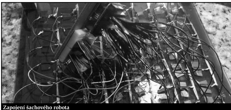
Zapojení šachového robota
